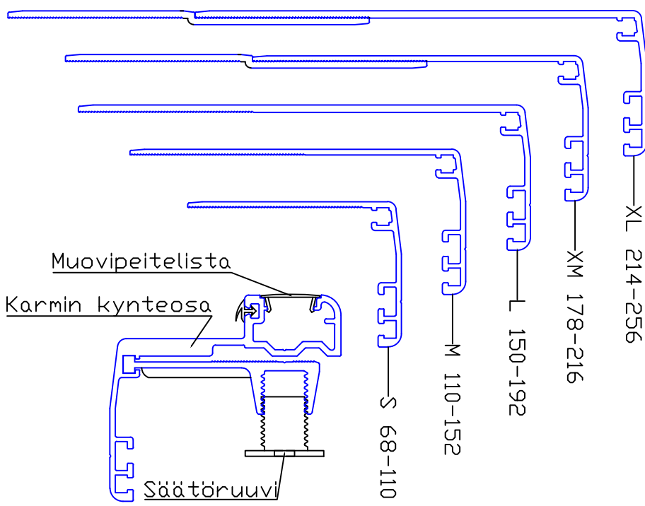
EI15/KAS 10
