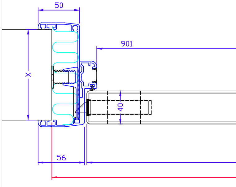
EI15/KAS 14 P
