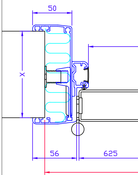
EI15/KAS 14 P
